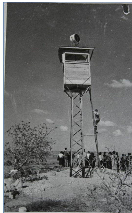
18. צילום ושרטוט חזיתות מגדל הפרוז'קטור (מקור: ארכיון קיבוץ ארז; ערכה: מסיקה 2017).
